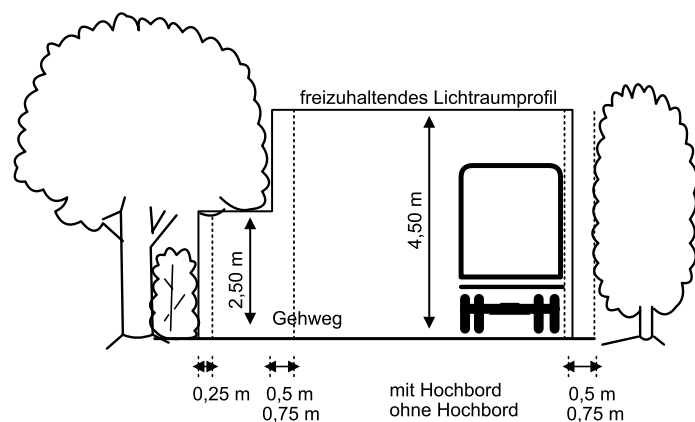
Abstände des freizuhaltenden Lichtraumprofils
